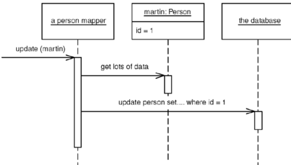
Figure 10.4. Updating data.
